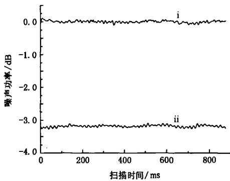
图3 测量到的强度差噪声 曲线 i SNL; 曲线 ii 强度差噪声
