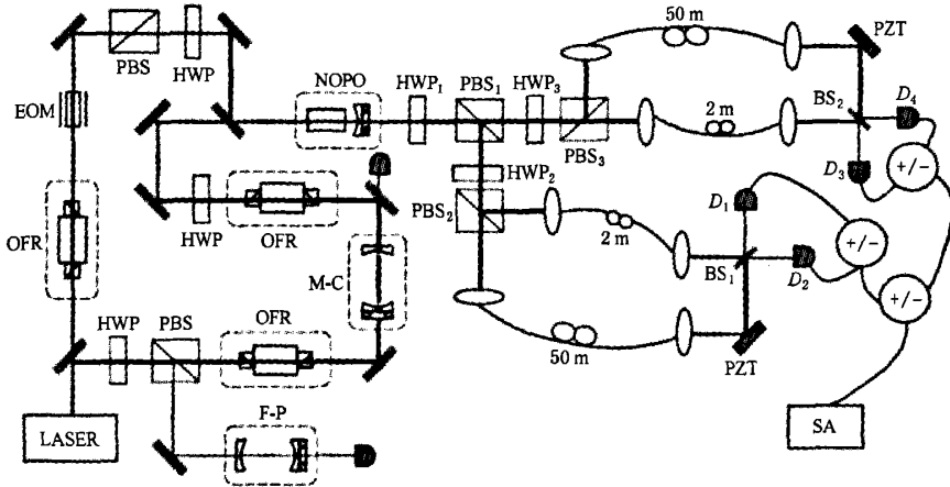
图2 制备高亮度频率非简并纠缠光场的实验装置(LASER为激光器;OFR为隔离器;F-P为Fabry-Perot腔;HWP为λ/2波片;PBS为偏振分束镜;EOM为电光调制器;M-C为模清洁剂;BS为分束片;PZT为压电陶瓷;D 1 -D 4 为光电探测器;+/-为加减法器;SA为频谱分析仪)
